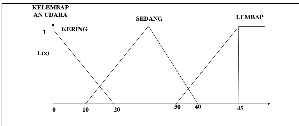
Gambar 4. 15 Kurva Kelembapan Udara.
